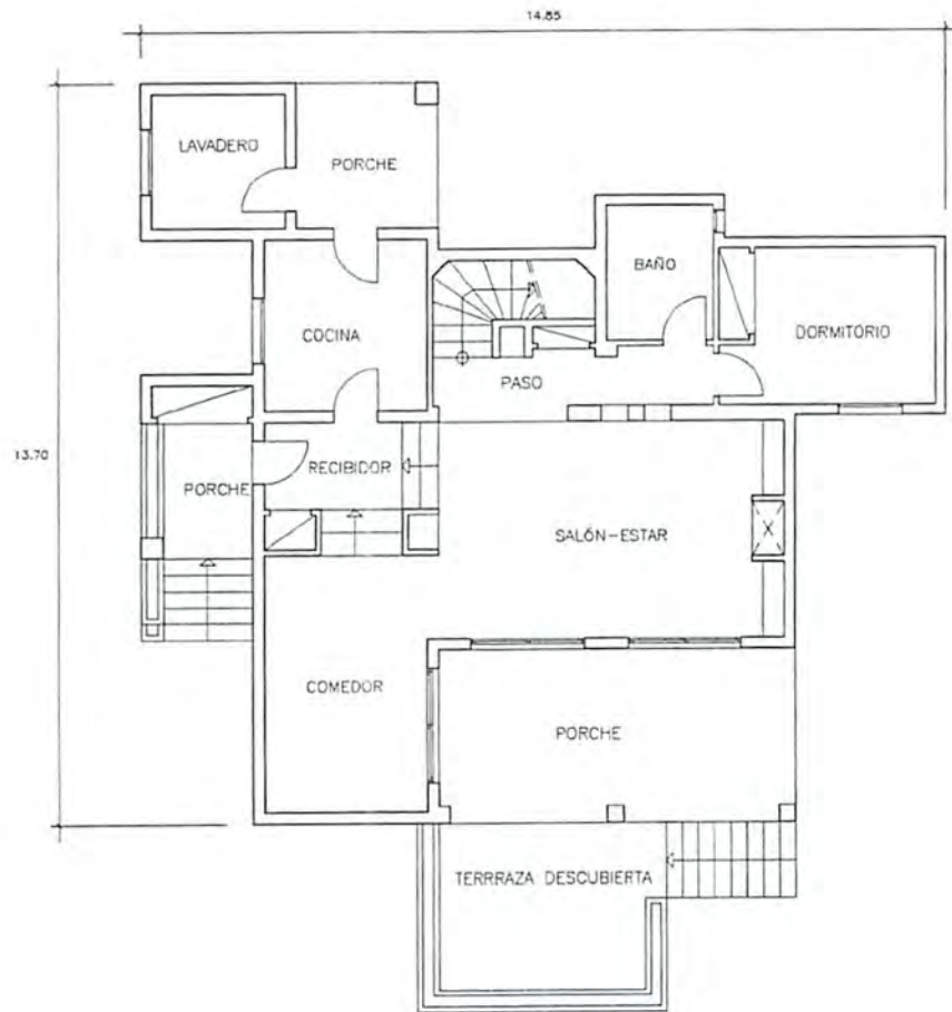
PLANTA BAJA
