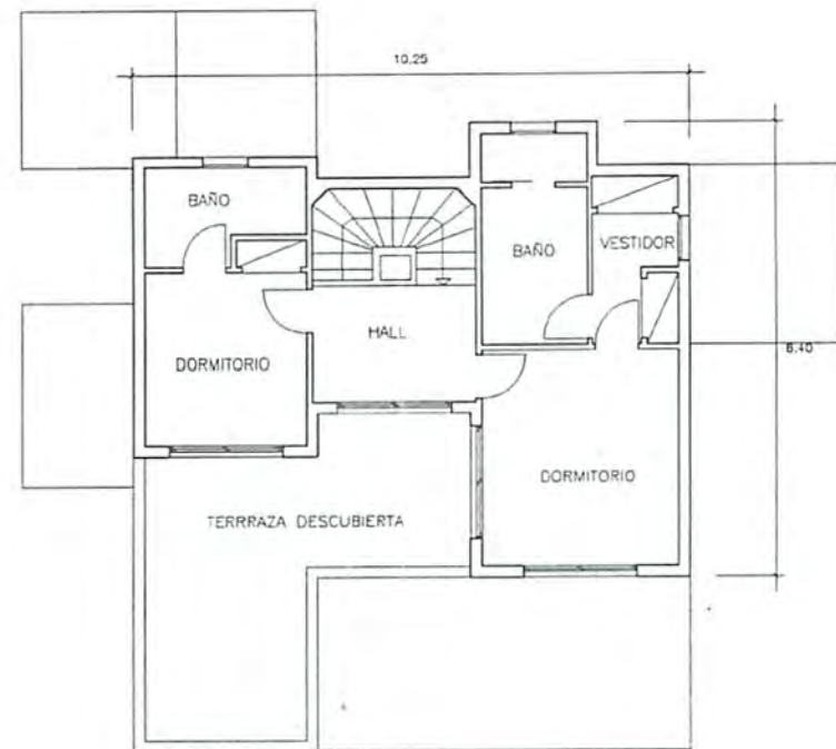
PLANTA PISO
